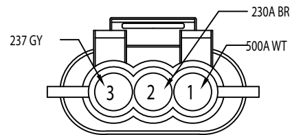
8.2/L LEFT STOP/TAILO 282087-1
