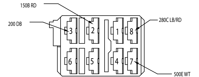
10.2 DOME LIGHT SWITCH (ETP) 999-16716-001
